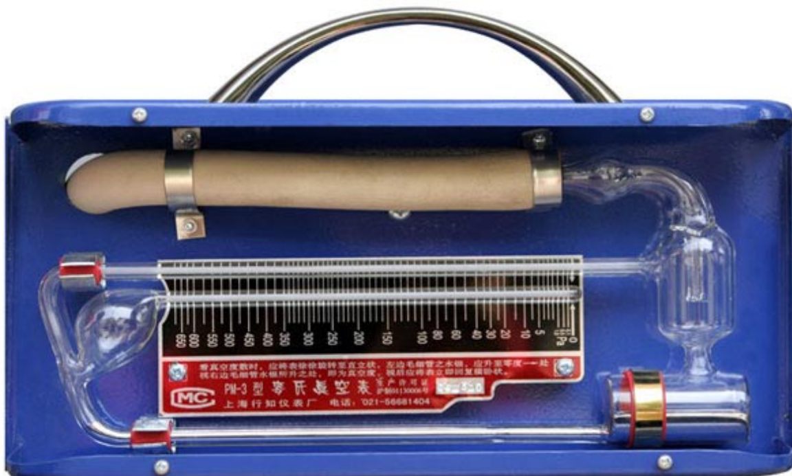
PM-3 流体型麦氏真空表 (测量范围 0.1Pa~650Pa)
