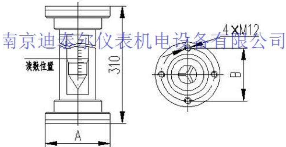
LZB-( )U型流量计外形图
