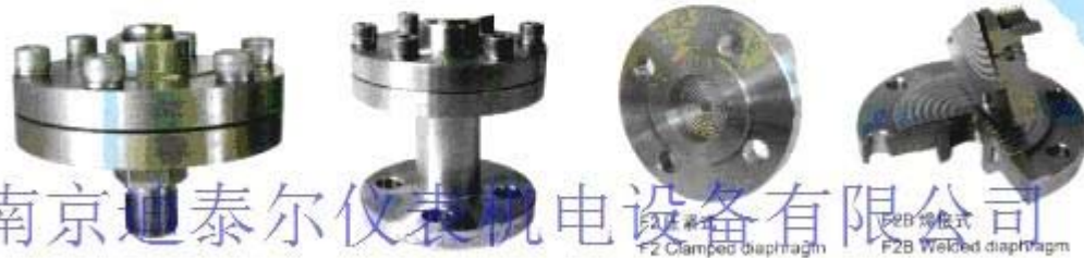
标准型 (不标代码) Standard type (without affix) | I型法兰 F1 F1 space flange | 敞开法兰 F2 F2 Open flange
