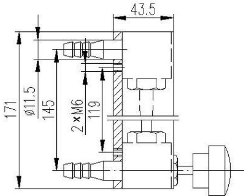
LZB-( )Q型流量计外形图
